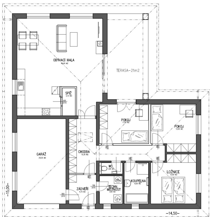
RODINNÝ DŮM RADEK Studie firmy FUTUR s.r.o.
